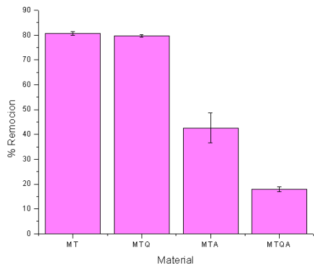
Figura 1. Porcentajes de remoción de omeprazol en los distintos materiales.
