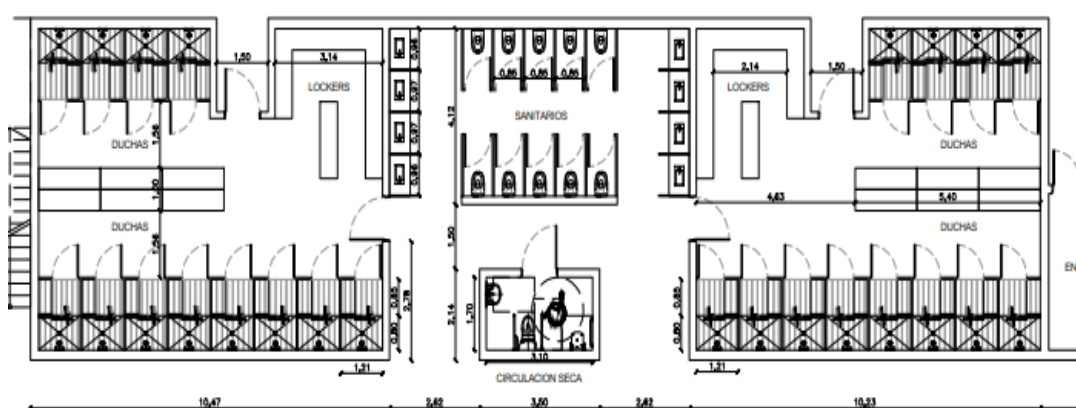
Figura 8: Sanitarios y vestuarios para atletas. Pileta Ciudad Deportiva.
