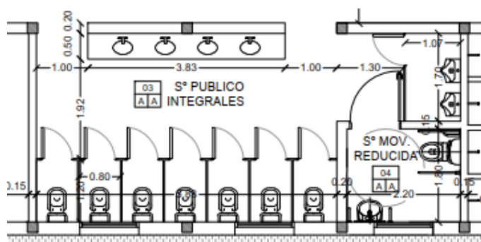
Figura 10: Sanitarios inclusivos para público en general. SAF.
