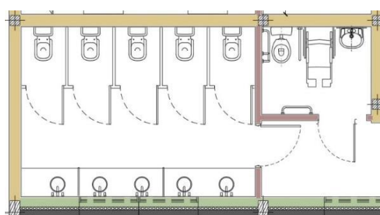
Figura 16: TOC. Sanitario Integral.
