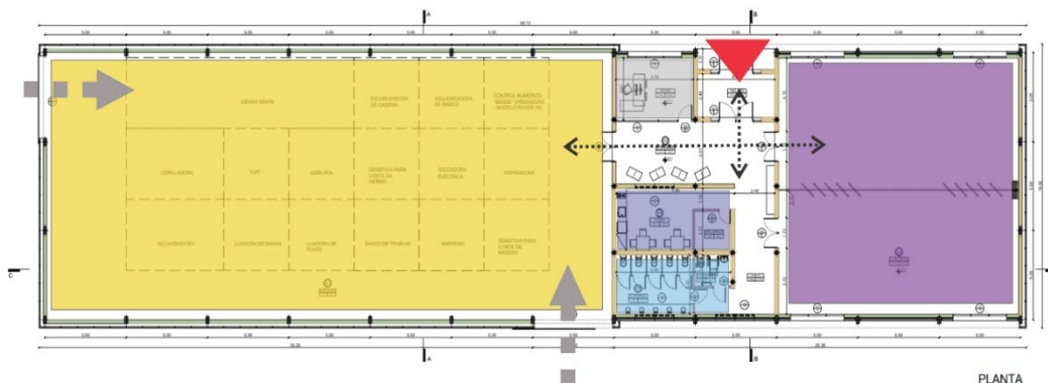
Figura 15: Organización funcional del conjunto: (rojo) acceso principal peatonal, (blanco) hall y circulación, (gris) oficina administrativa, (azul) cocina comedor, (celeste) sanitario integral, (amarillo ocre) carpintería y (violeta) talleres de oficio.
