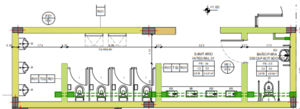
Figura 4: Sanitarios PB EMA para público en general.
