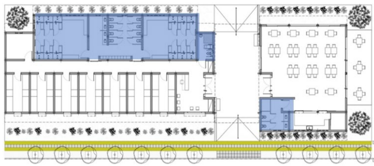
Figura 19: Planta General del Albergue y Comedor del Complejo Deportivo Recreativo, a la derecha se encuentra el sector de albergue con vestuarios, sanitarios integrales, y modulo sanitario completo inclusivo; a la izquierda el comedor con sanitarios integral.
