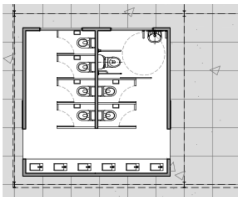
Figura 6: Sanitarios Paseo de Artesanos, proyecto CAUr
