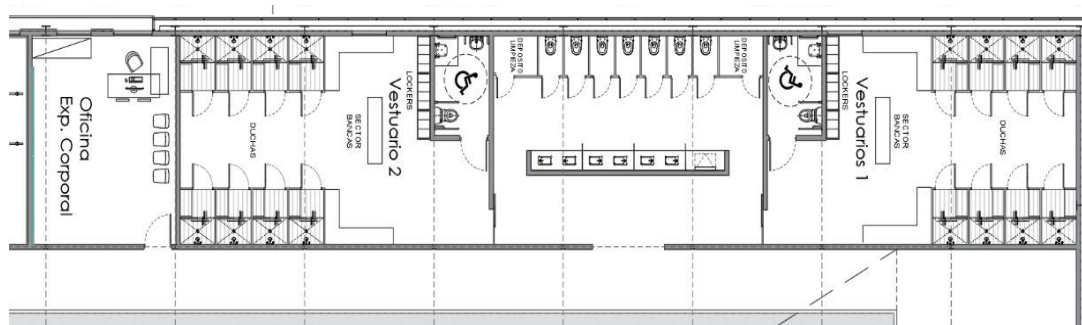
Figura 14: CEPAP Organización Funcional de Sanitarios y Vestuarios Integrales en planta baja.
