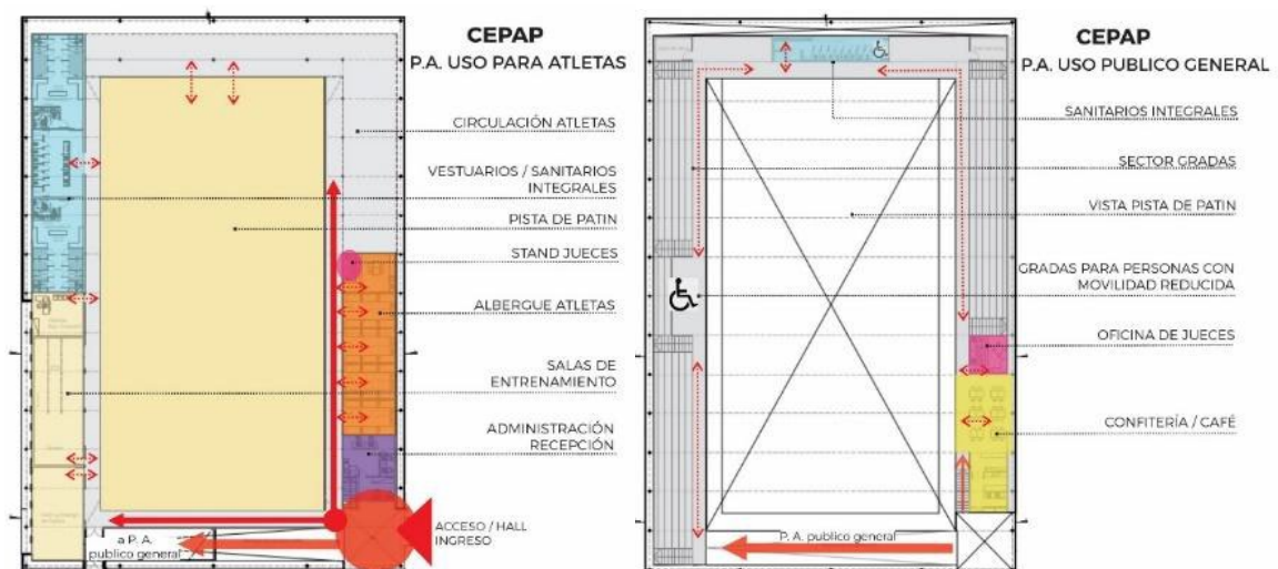
Figura 12: Organización funcional de CEPAP. P.B. Uso para atletas y P.A. uso público en general
