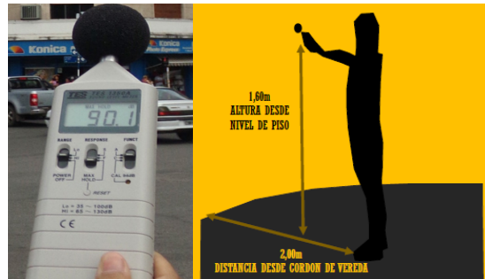
Figura 6. Sonómetro. Protocolo de Medición
