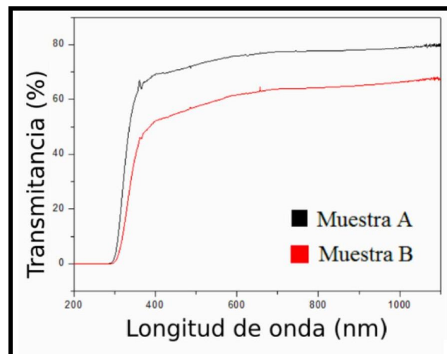
Figura 2. Comparación de los espectros de transmisión de la Muestra A y Muestra B.
