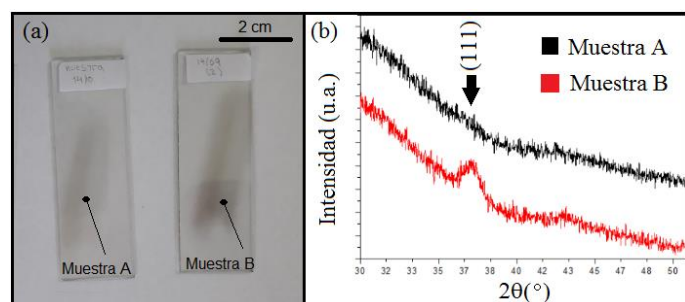
Figura 1(a). Imágenes macroscópicas de films de NiO obtenidos (b) Medida de difractograma de rayos X en los films.
