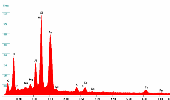
Figura 3: EDX de sector con cianolíquenes. Se observa el pico de C y O en concordancia con la actividad biológica.
