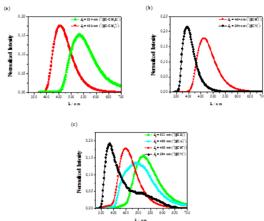
Figura 2. Intensidad de emisión de fluorescencia normalizada de los espectros obtenidos con el análisis paralelo de factores (PARAFAC) de la titulación ácido-base de una solución acuosa alcalina de: (a) 2-Ma-nHo, (b) 9-Ma-nHo, y (c) nHo
