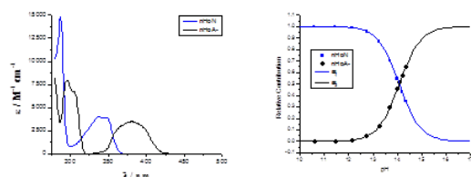
Figura 1. Contribución relativa vs pH (derecha) y absorptividad molar optimizada (izquierda) de las especies deconvolucionadas presentes en el equilibrio de disociación ácida ( K_a ) del nitrógeno indólico (N-9) de nHo, obtenido por la metodología de modelado MCR-ALS híbrida (duro blando).
