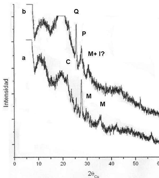
Figura 5. DRX comparativo de material oscuro (tamaño 3 mm) con diferente contenido de cristaloclastos. (P: plagioclasa, Q: cuarzo, C: cristobalita, M: magnetita, I: ilmenita)
