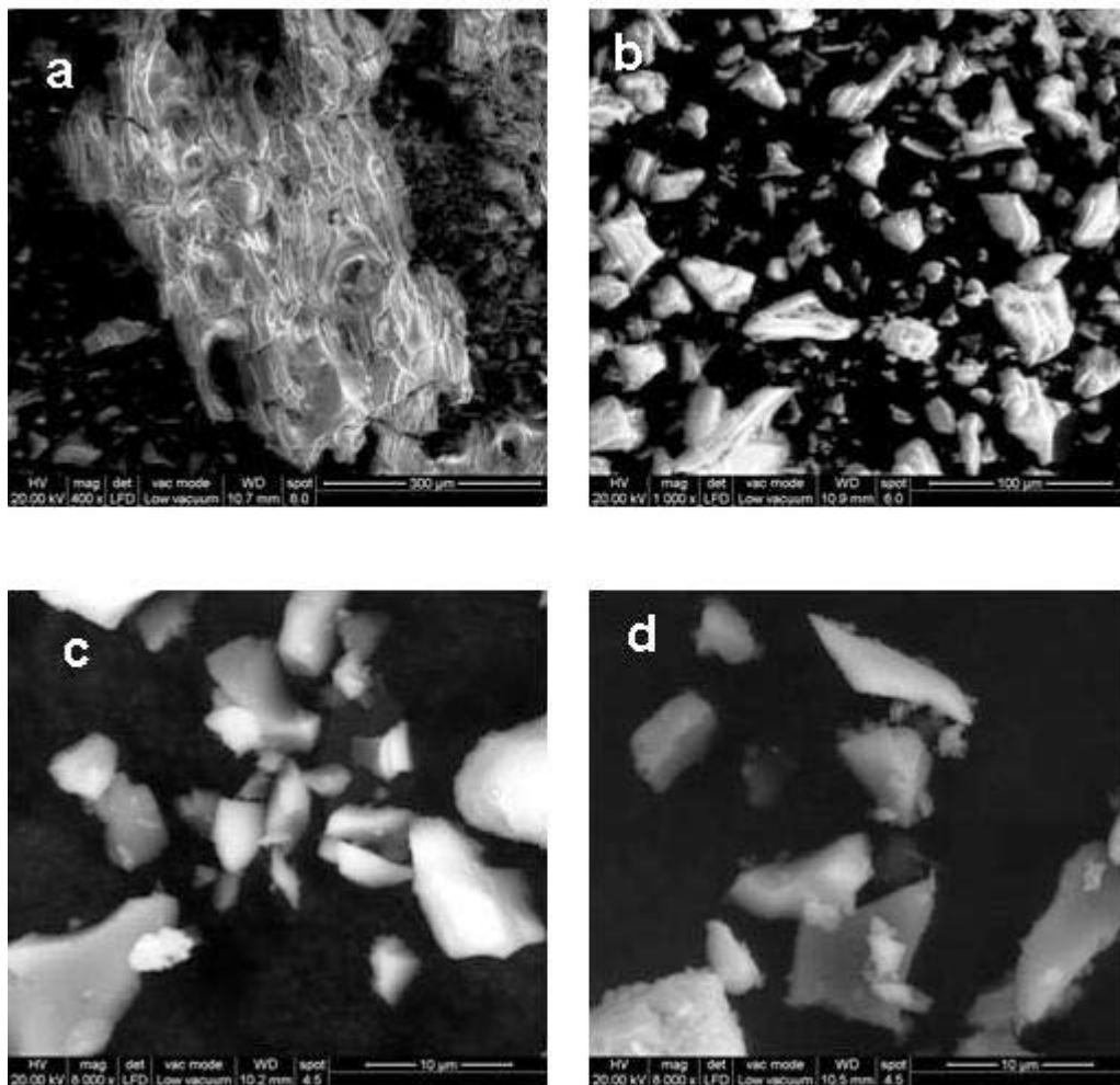
Figura 6. Micrografías SEM de material fino a diferente magnificación: a) eventuales partículas de tamaño superior a 100\ \mu\text{m} , x 400, b) x 1000, c) y d) x 8000.
