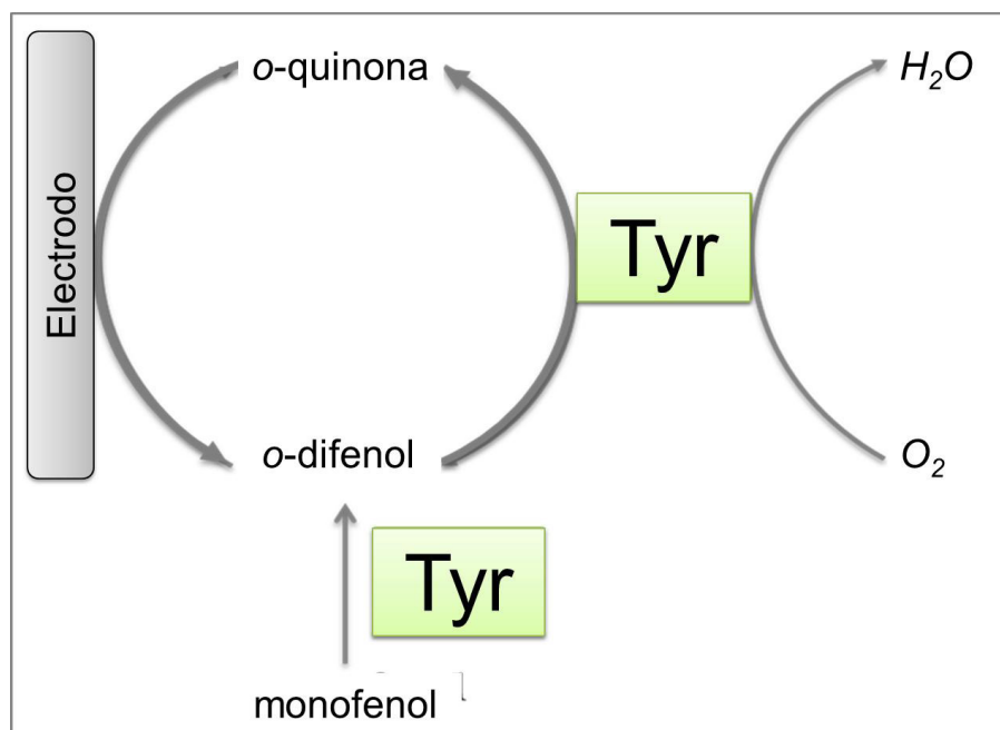
Figura 2. Reacción global del biosensor de Tirosinasa para la detección de fenoles.
