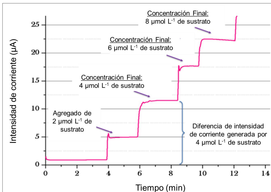
Figura 4. Amperograma obtenido con el biosensor de Tirosinasa a distintas concentraciones de catecol (adiciones sucesivas de 0 a 8 \mu\text{mol L}^{-1} ). Condiciones de trabajo (ver en texto).
