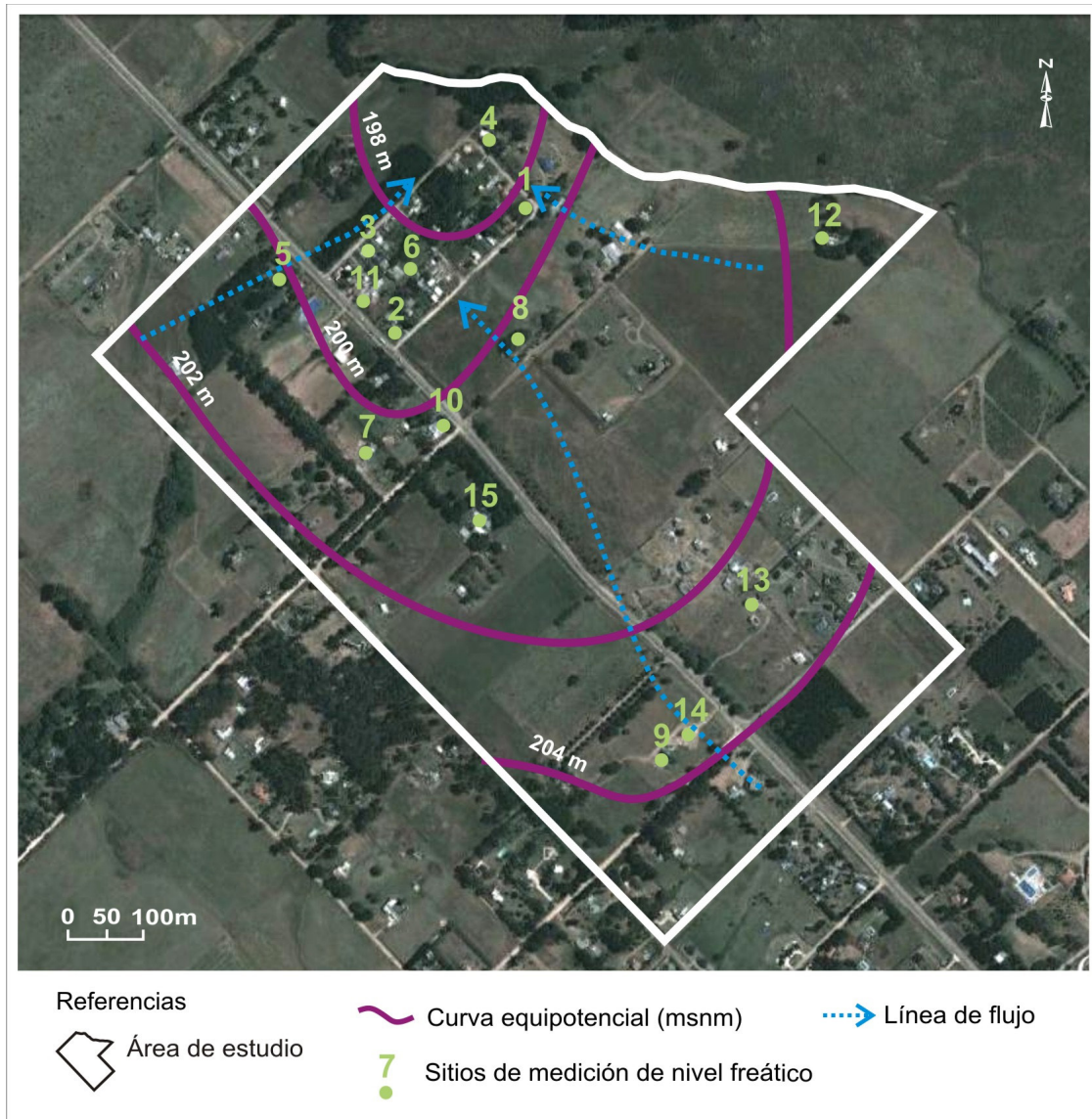
Figura 4. Mapa equipotencial para junio 2011.
