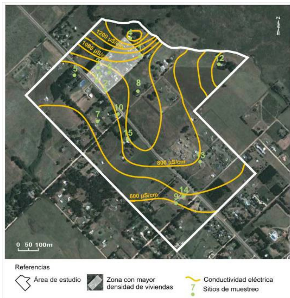
Figura 5. Mapa de isoconductividad (febrero 2011).
