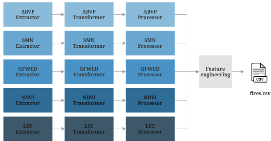
Fig. 1. Arquitectura conceptual del pipeline de datos.
