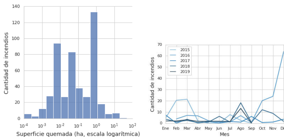
Fig. 4. Cantidad de incendios según magnitud (izquierda) y según el mes y año (derecha).
