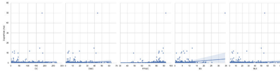
Fig. 6. Relación entre la superficie quemada en hectáreas por incendios forestales y los componentes del índice meteorológico de peligro de incendio.
