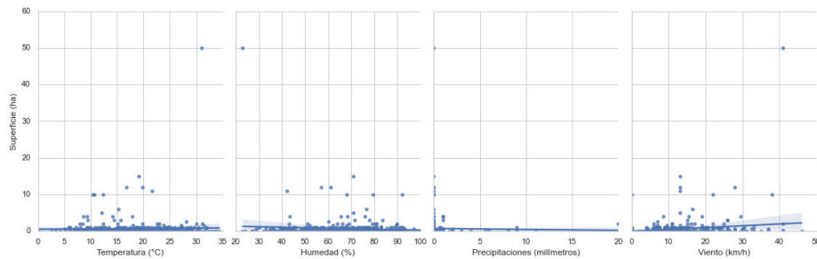
Fig. 5. Relación entre la superficie quemada en hectáreas por incendios forestales y distintas variables climáticas.
