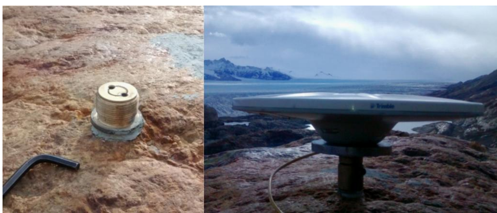
Figura 1. Monumentación con anclaje de posición fija. Figure 1. Stainless Steel Mast.
