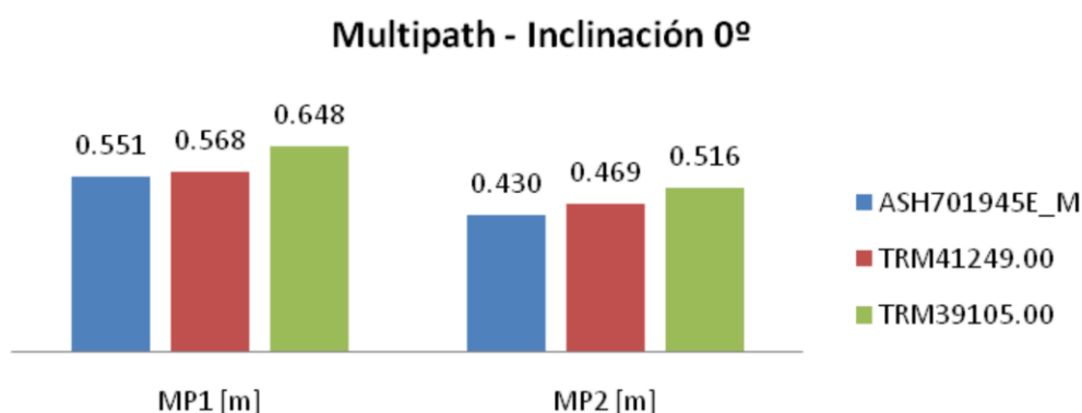
Figura 6. Multipath estimado de las 3 antenas con inclinación 0°. Figure 6. Estimated multipath of the 3 antennas with tilt 0°.
