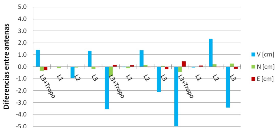
Figura 9. Comparación de posiciones entre las antenas con inclinación 0^\circ .
